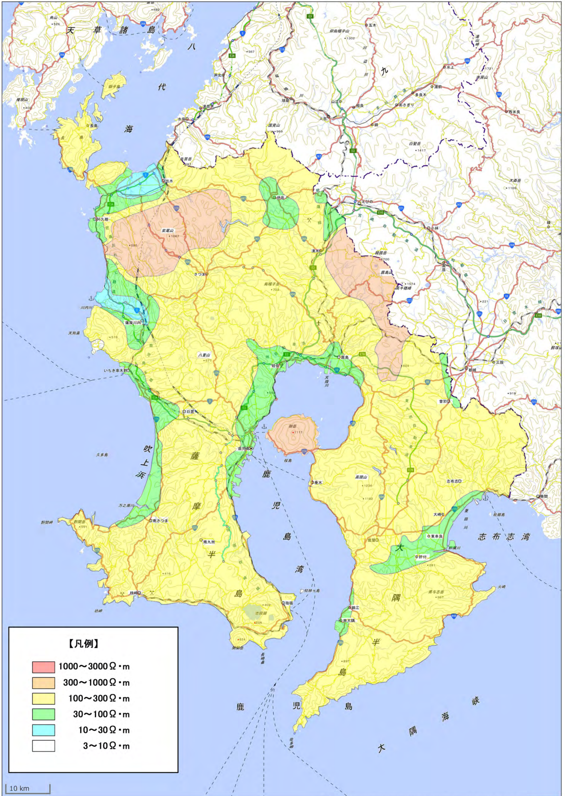
鹿児島県の大地抵抗率図
