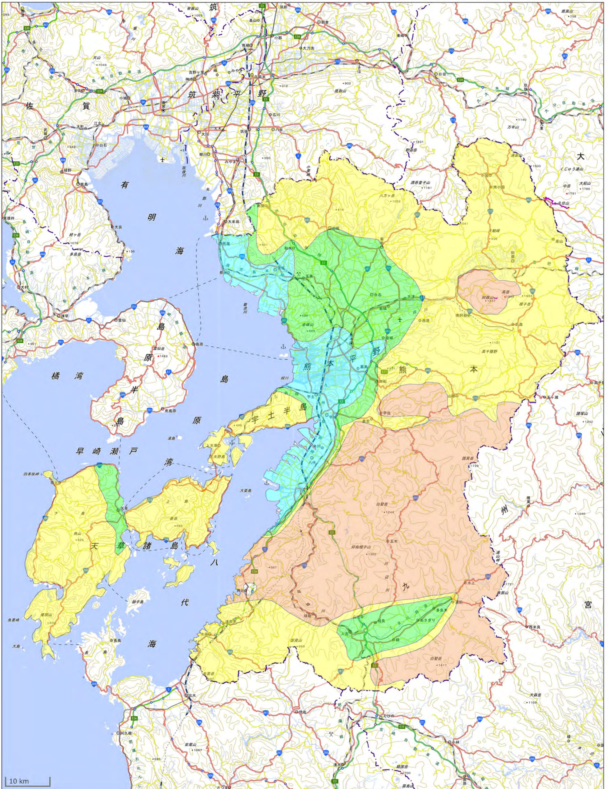
日本の大地導電率（1969）：電気学会・電子通信学会から引用・加筆 地図は地理院地図（電子国土Web）を使用した
