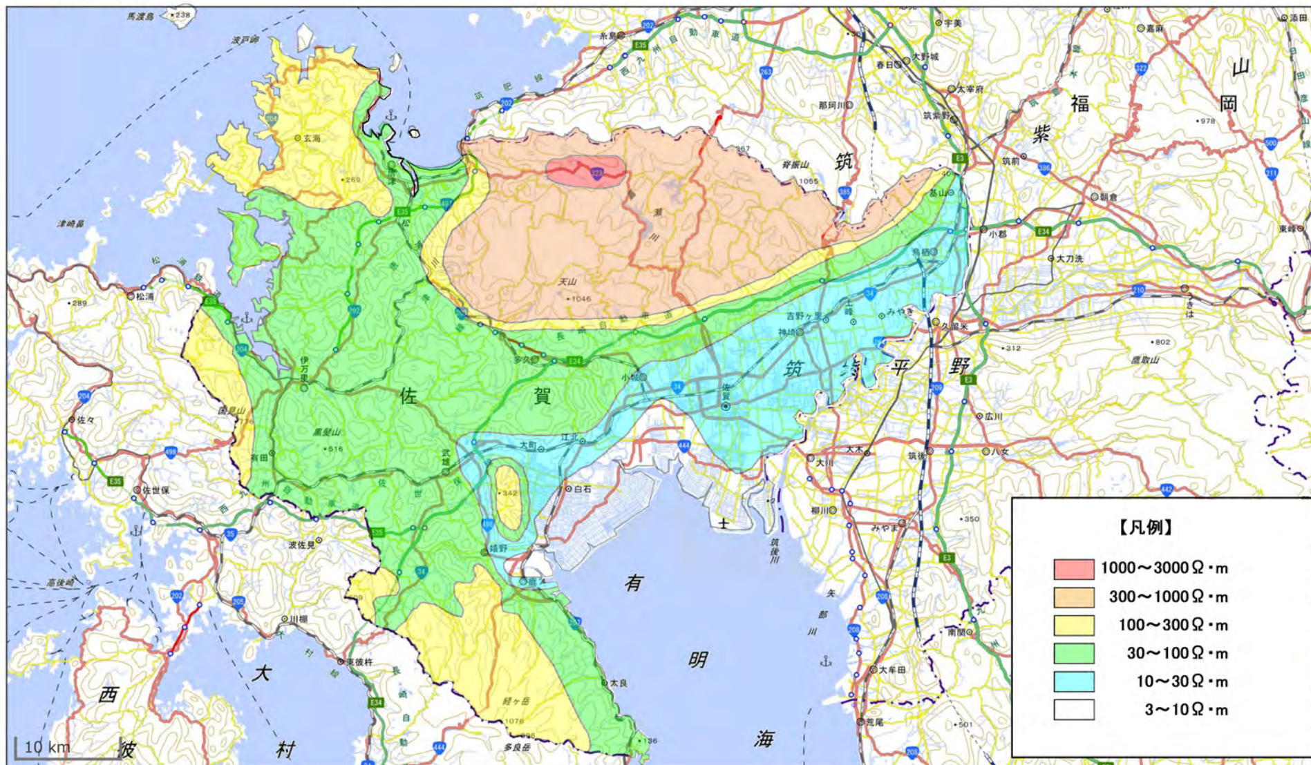
佐賀県の大地抵抗率図
