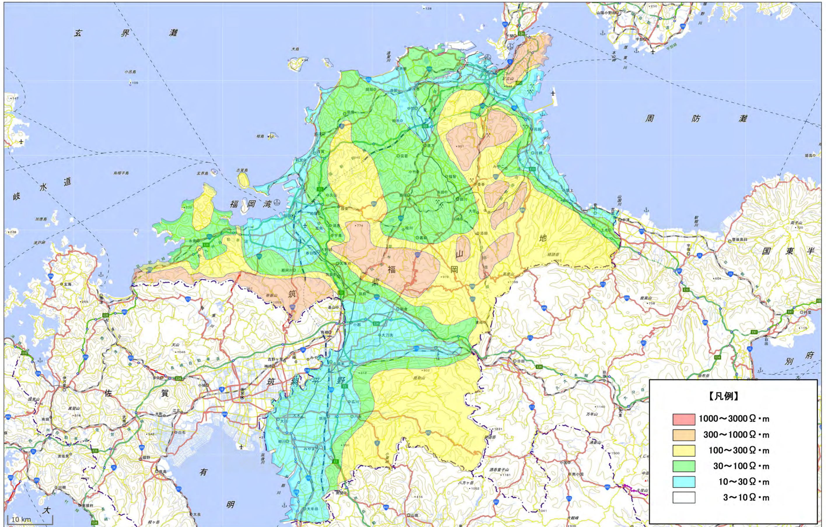
日本の大地導電率（1969）：電気学会・電子通信学会から引用・加筆 地図は地理院地図（電子国土Web）を使用した 福岡県の大地抵抗率図
