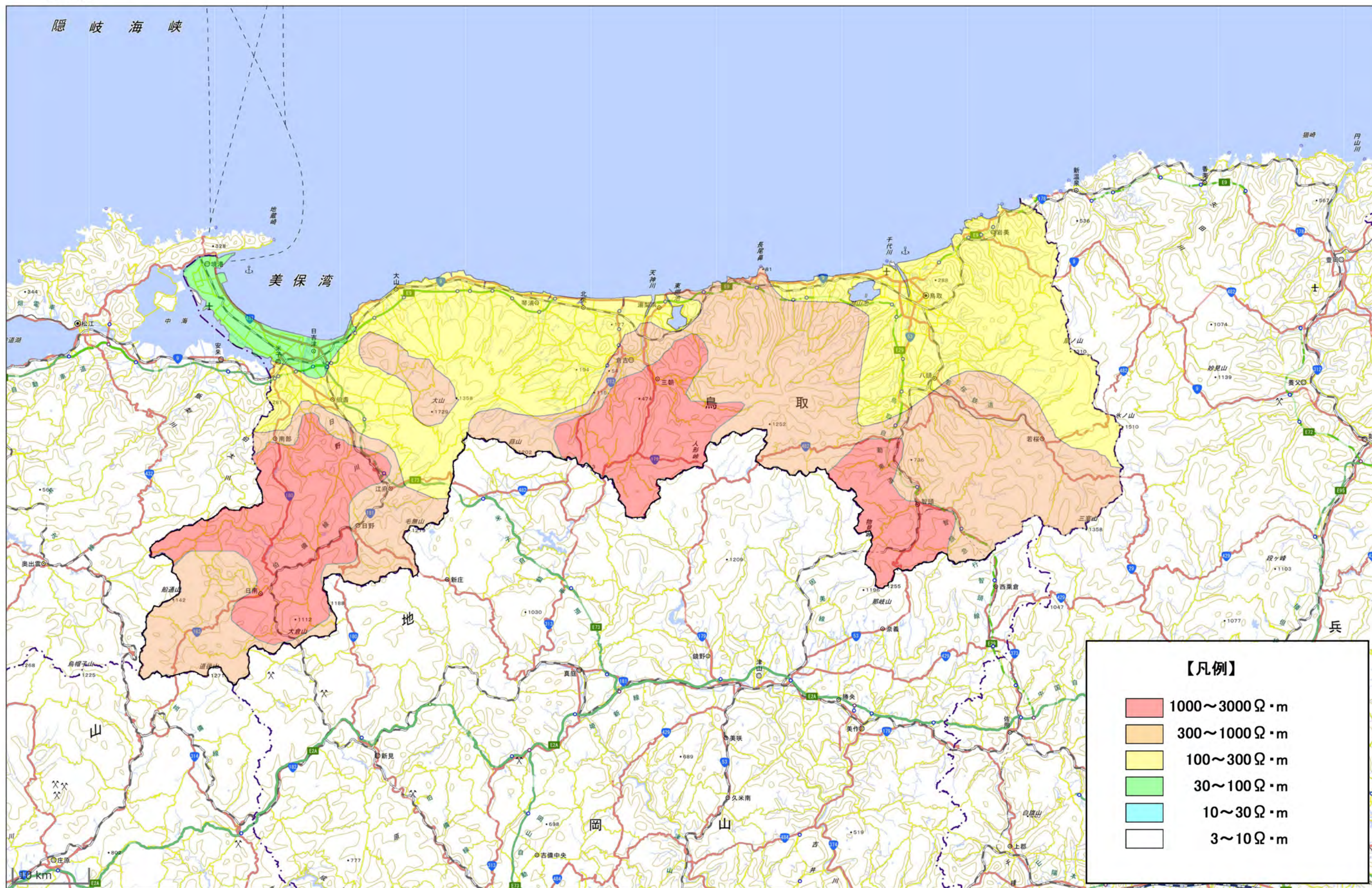
日本の大地導電率（1969）：電気学会・電子通信学会から引用・加筆 地図は地理院地図（電子国土Web）を使用した
