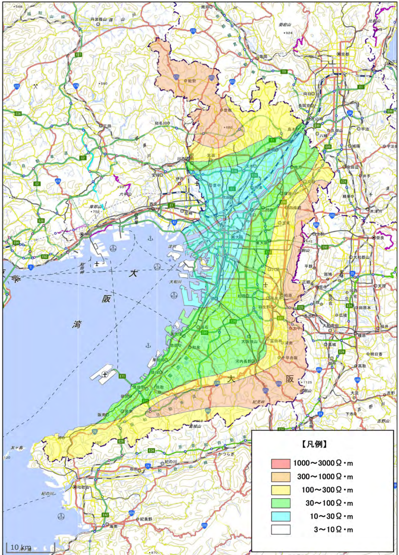
日本の大地導電率（1969）：電気学会・電子通信学会から引用・加筆 地図は地理院地図（電子国土Web）を使用した 大阪府の大地抵抗率図
