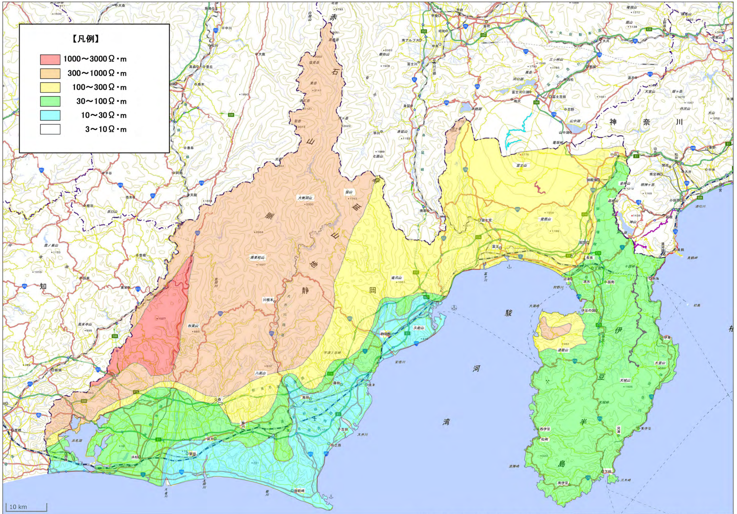
日本の大地導電率（1969）：電気学会・電子通信学会から引用・加筆 地図は地理院地図（電子国土Web）を使用した
