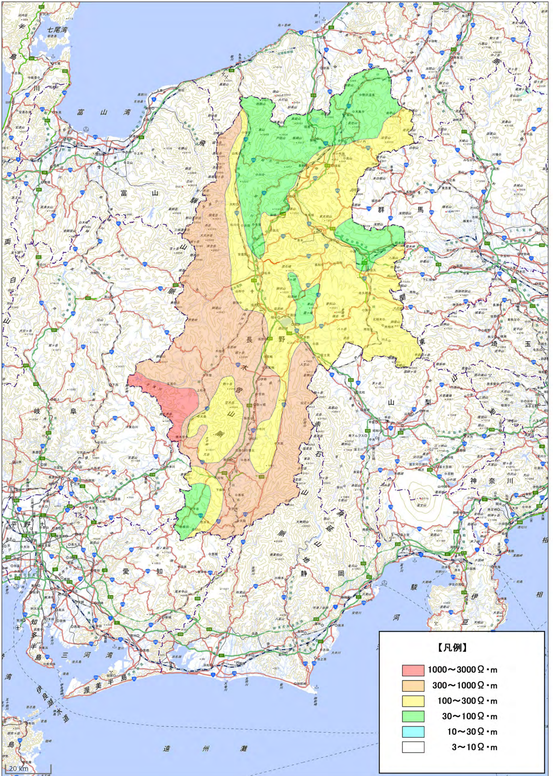
日本の大地導電率（1969）：電気学会・電子通信学会から引用・加筆 地図は地理院地図（電子国土Web）を使用した 長野県の大地抵抗率図
