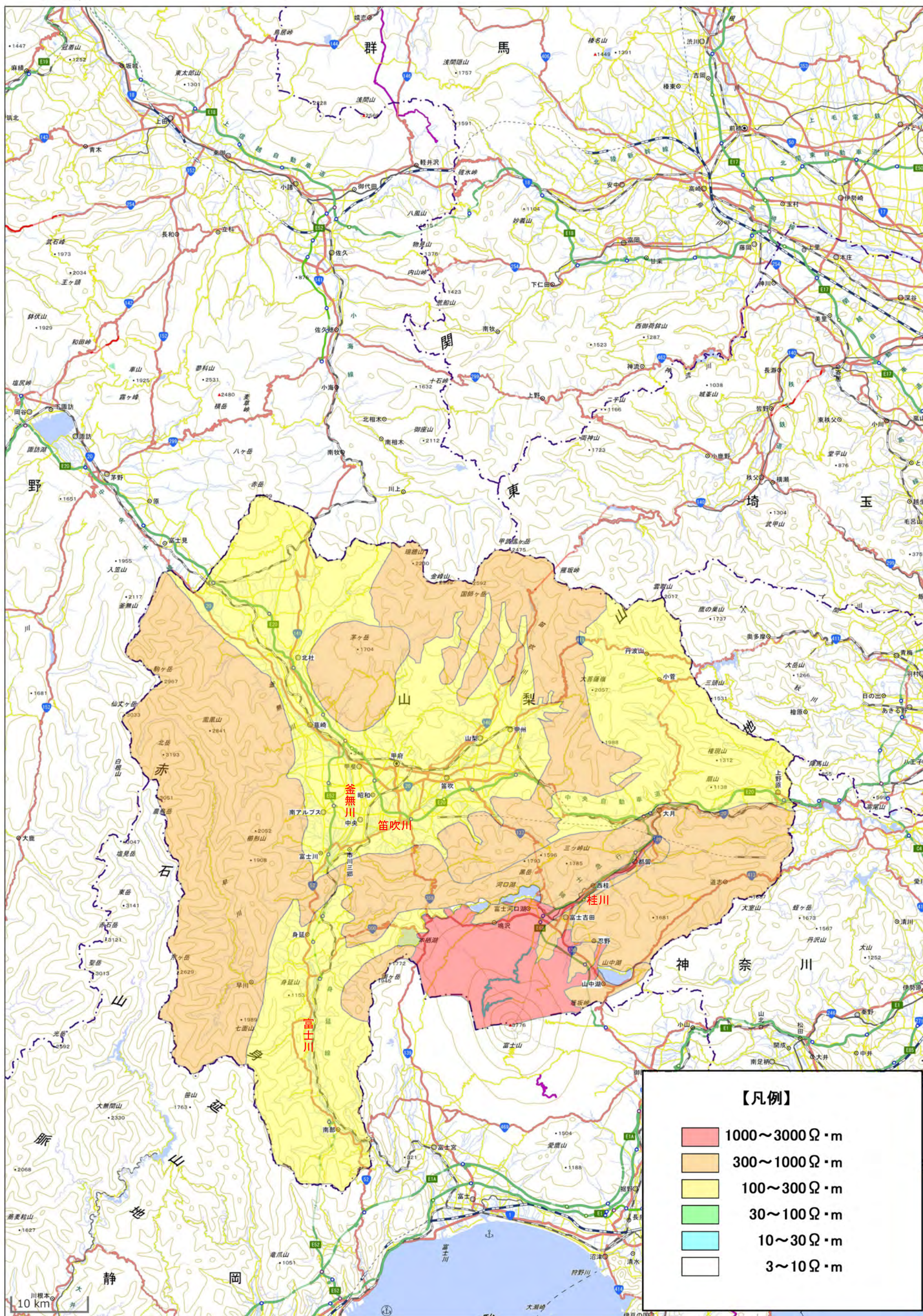
山梨県の大地抵抗率図
