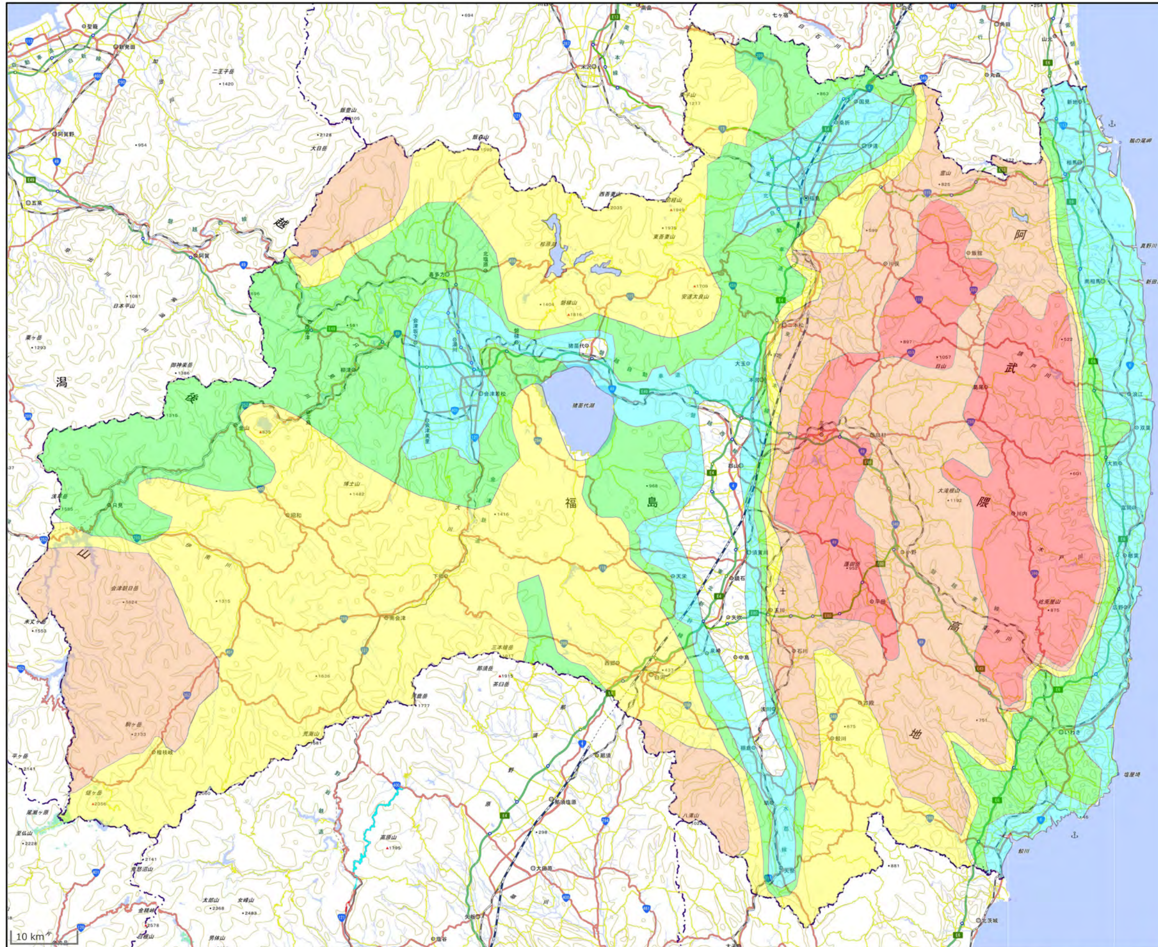
日本の大地導電率（1969）：電気学会・電子通信学会から引用・加筆 地図は地理院地図（電子国土Web）を使用した
