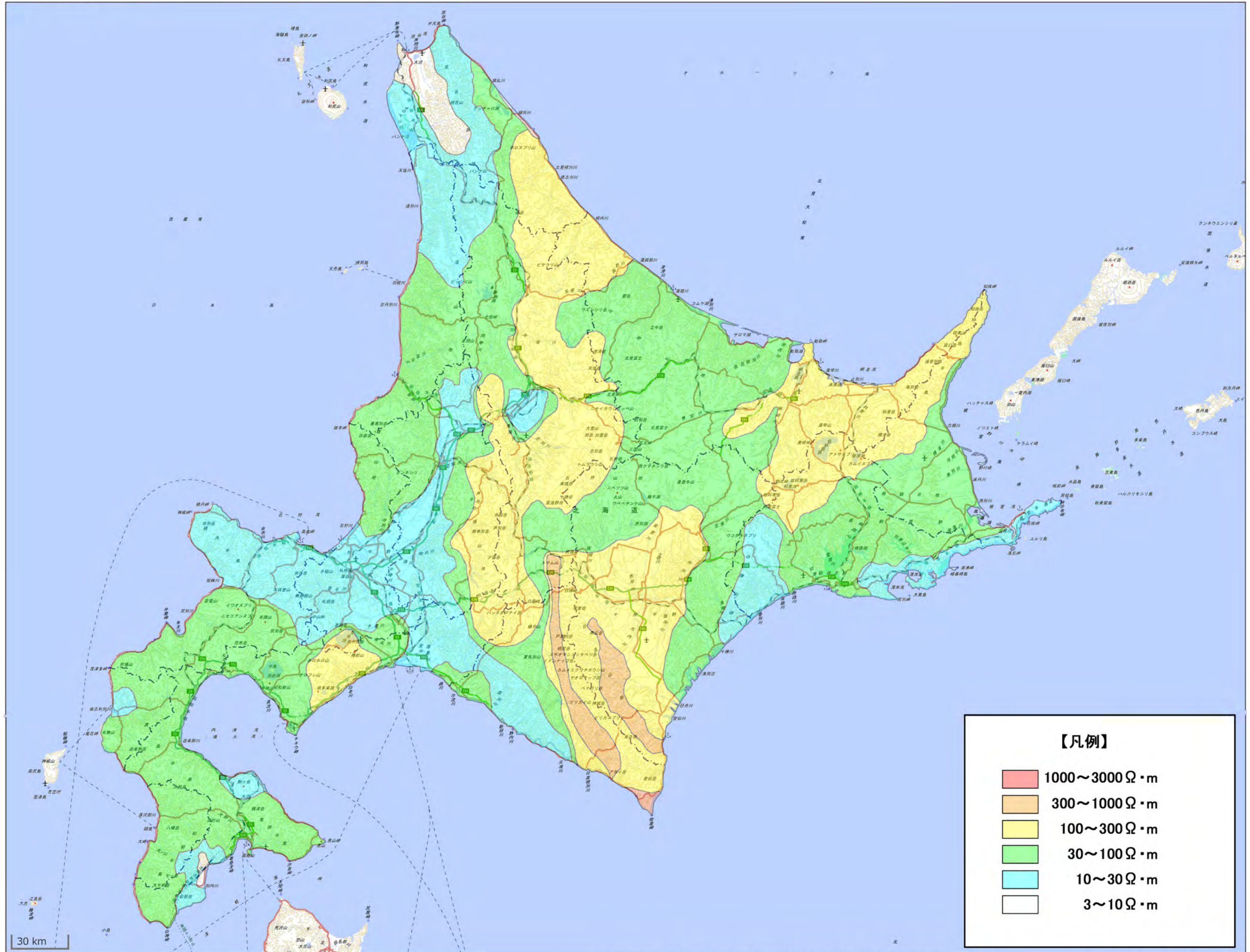
日本の大地導電率（1969）：電気学会・電子通信学会から引用・加筆 地図は地理院地図（電子国土Web）を使用した
